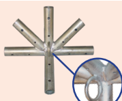
6-punktowy trójkąt boczny z pierścieniem F116WSTRING
